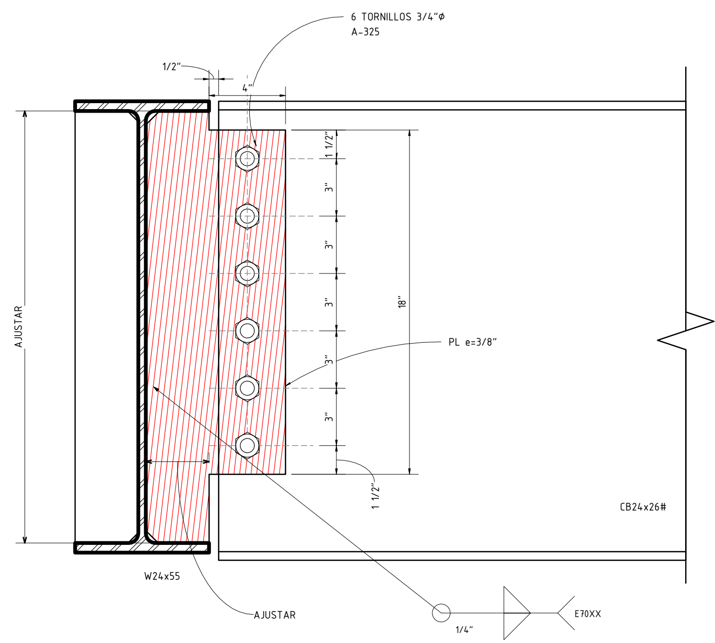
1 CONEXION CB24x26 A TRABE W24x55 Section 1:5
