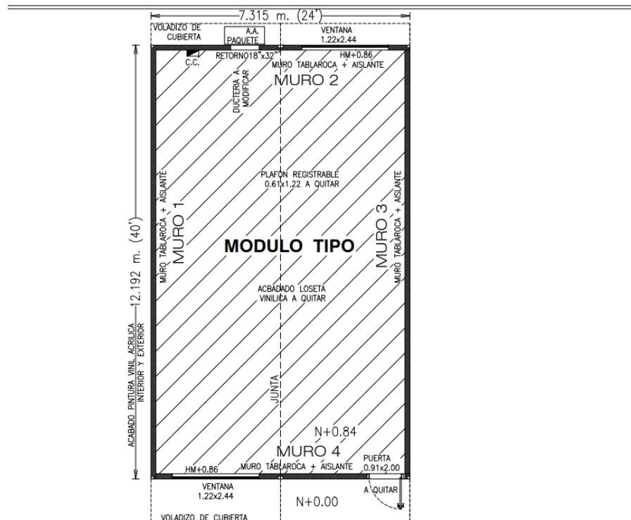
MODULO MOVIL TIPO DE 24'(7.315 M.) x 40'(12.192 M.) DESPLANTADOS E INTEGRADOS EN SITIO AUN SIN MODIFICAR
